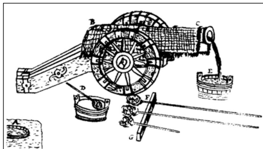
Рис. 7. Охлаждение орудия после стрельбы. Гравюра конца XVII в.
